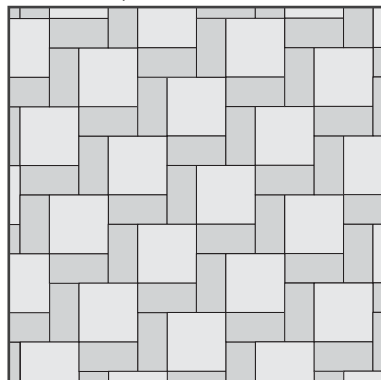
VZOR PDN 7 / DLAŽBA TAĹÁNA
