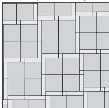
VZOR PDN 11 / DLAŽBA VIVIAN, BIANCA
