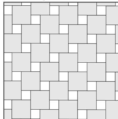
VZOR PDN 1-1 / DLAŽBA TAĀTĀNA
